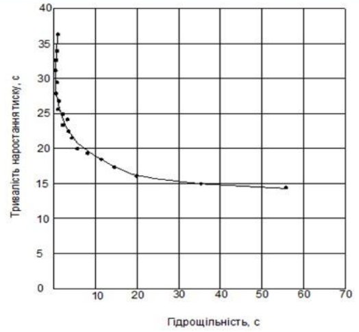
Залежність тривалості наростання тиску від гідроцильності плунжерних пар
