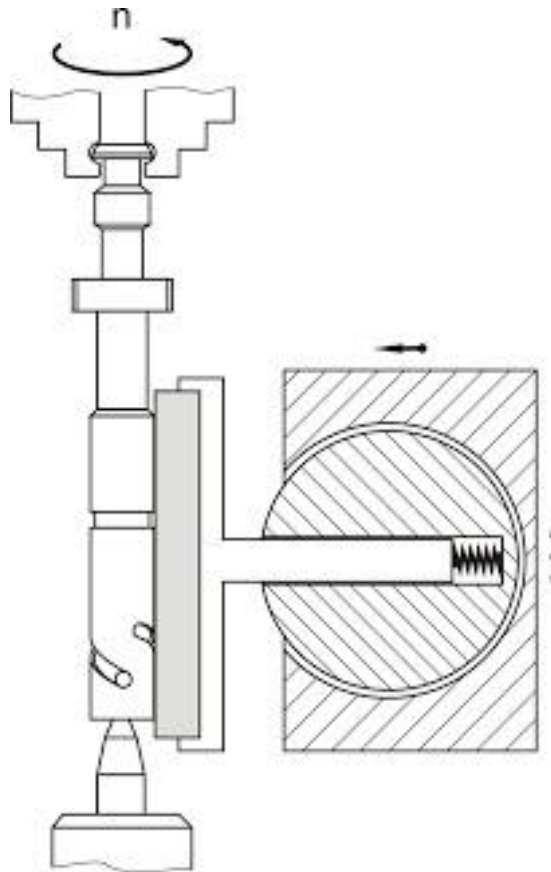
Рис.2.6. Схема пристрою для шліфування поверхні плунжера
