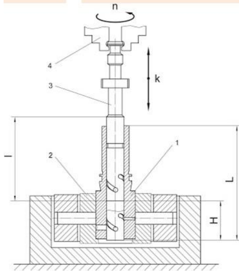
Схема спільного перешліфування зношених робочих поверхонь плунжера й гільзи
