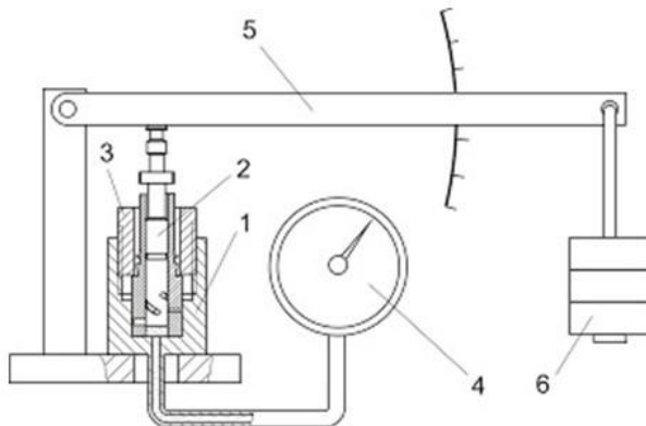
Схема станда для контролю гідравлічної щільності плунжерних пар
