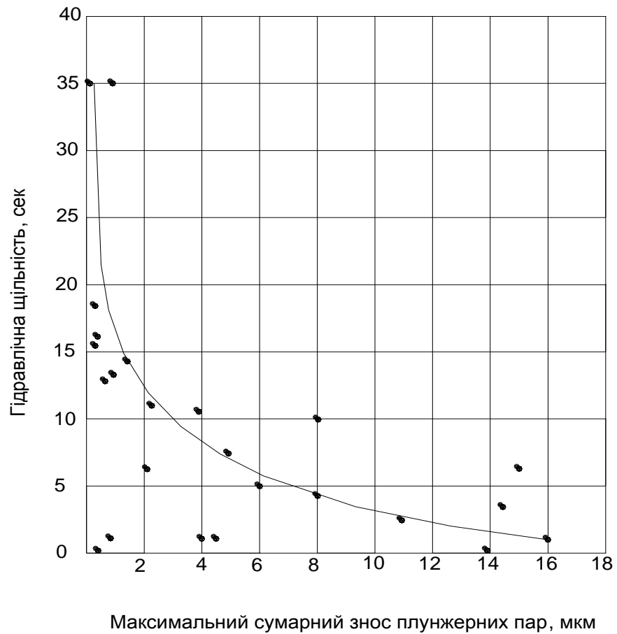
Рис.3.13. Залежність гідрощільності плунжерних пар від їх максимального сумарного зношування
