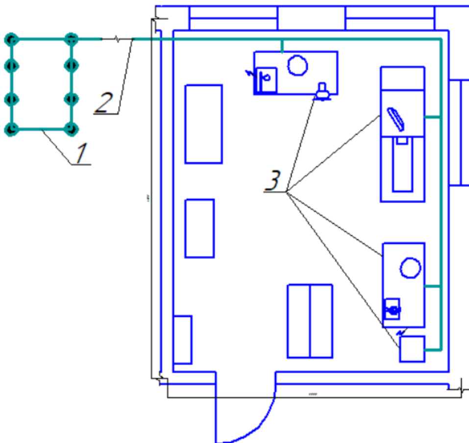
Рис. 4.1. Схема заземлення паливної дільниці
