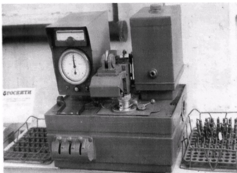
Рис. 3.3. Прилад КИ-3369 для випробувань плунжерних пар на гідроцільність.
