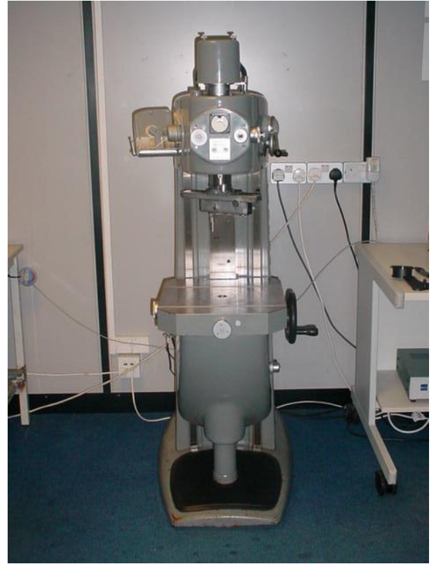
Рис.3.1. Профілограф «Talyurf» для дослідження мікро геометрії плунжерних пар
