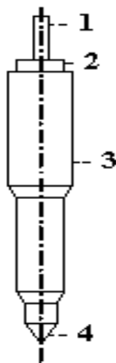
Рис. 1.6. Місця зношення поверхні голки
