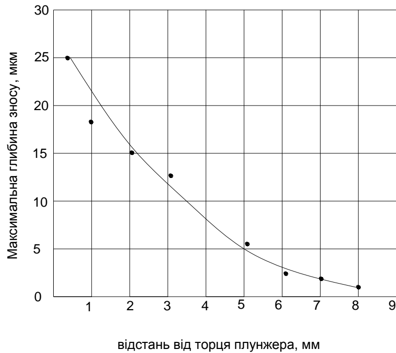
Рис. 3.11. Глибина зношування плунжера ЯЗТА залежно від відстані від торця
