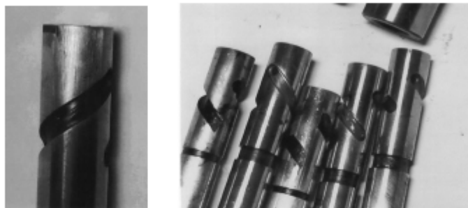
Рисунок 1. Зовнішній вигляд зношених плунжерів: а - ЯМЗ, б – УТН
