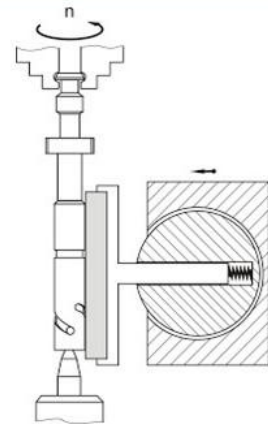
Схема пристрою для шліфування поверхні плунжера
