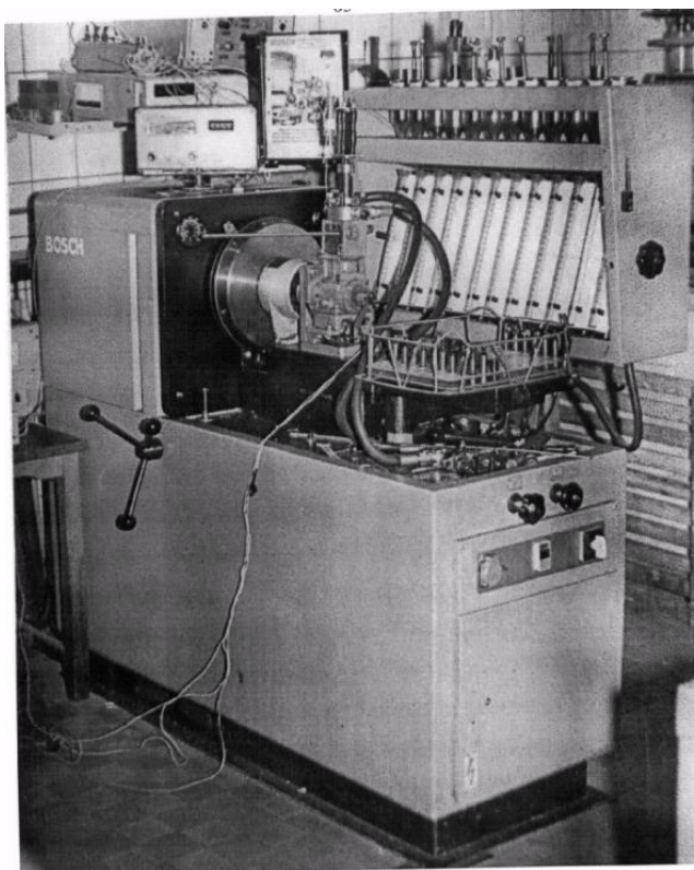
Рис. 3.7. Контрольно - регулювальний стенд « Bosch » для безмоторних досліджень плунжерних пар.
