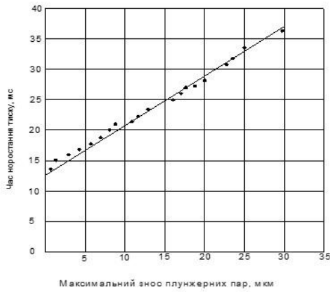
Залежність часу наростання тиску від максимального зносу плунжерних пар
