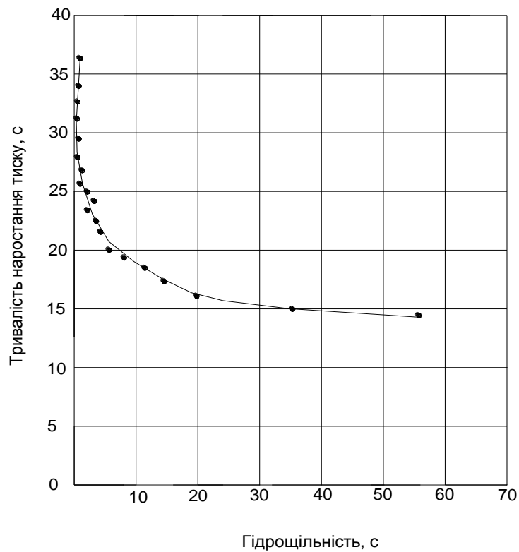
Рис.3.16. Залежність тривалості наростання тиску від гідроцільності плунжерних пар
