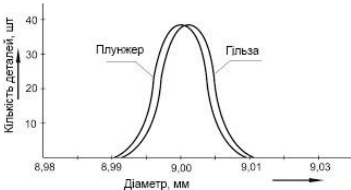
Рис 2.3. Розподіл розмірів плунжера й гільзи до перешліфування
