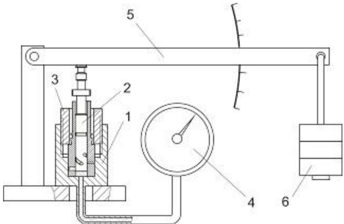
Рис.2.8. Схема стенда для контролю гідравлічної щільності плунжерних пар
