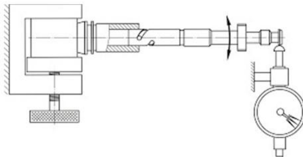
Схема пристрою для визначення величини зазору в плунжерній парі по розмахові хитання плунжера
