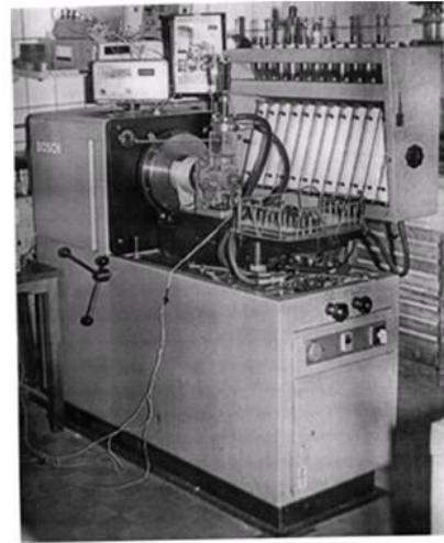
Контрольно - регулювальний стенд « Bosch » для безмоторних досліджень плунжерних пар
