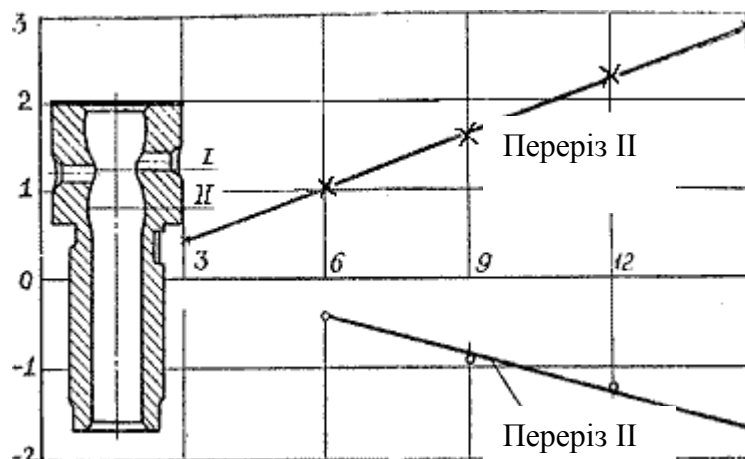
Рис.1.4. Зміна величини зазору плунжерної пари залежно від зусиль затягування
