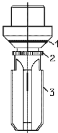
Рис. 1.5. Поверхні нагнітаючого клапана, що підлягають зносу 1-запирний конус; 2-розвантажувальний поясок; 3-направний хвостовик
