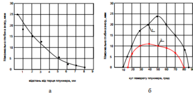
Рисунок 2. Глибина зношування плунжера та її зміна а - глибина зношування плунжера ЯЗТА залежно від відстані від торця, б - зміна глибини зношування плунжера ЯЗТА залежно від кута повороту 1 – зношування на відстані 0,5 мм від торця плунжера 2 – зношування на відстані 3 мм від торця плунжера
