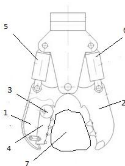
Рис.1 Гидрожницы с эксцентриковым механизмом / Hydraulic shears with an eccentric mechanism
