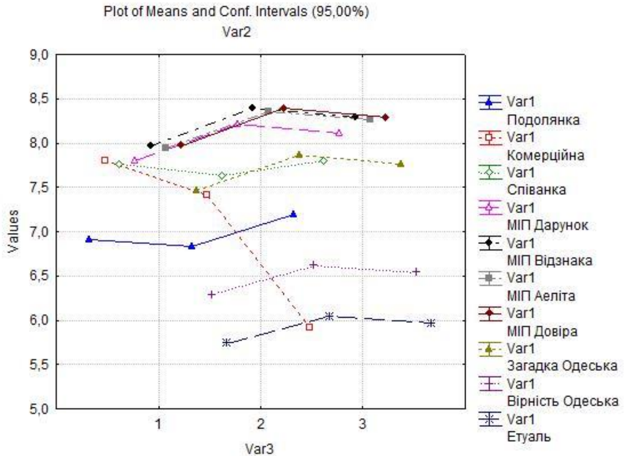
Рис. 3. Генотип-середовищна взаємодія.
