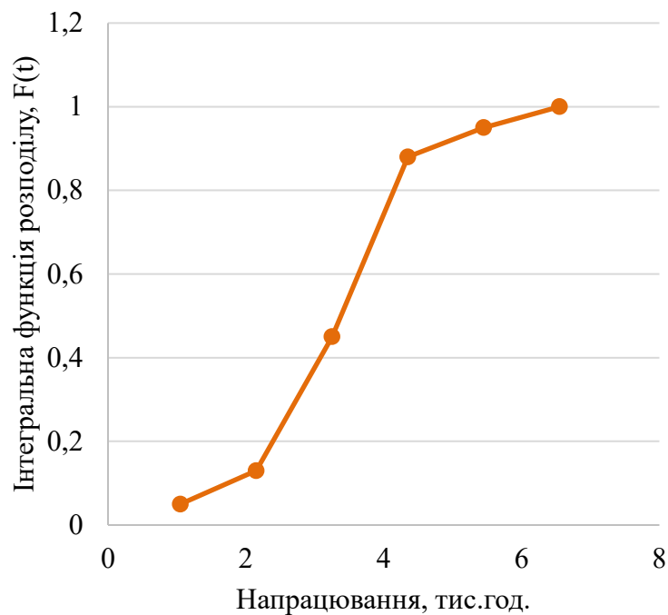
Рисунок 3.13 - Інтегральна функція наробітку комбайнів
