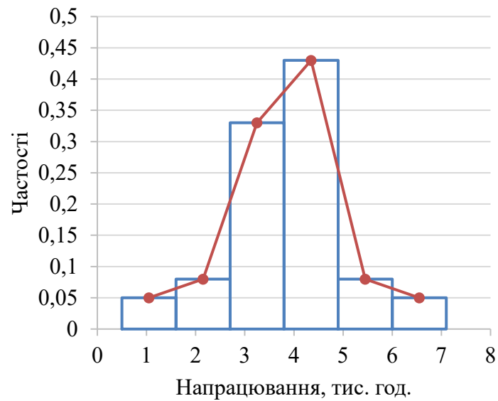
Рисунок 3.12 - Зображення гістограми та полігона в загальному вигляді
