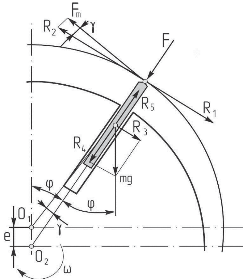
Рис. 3. Схема сил, які діють на пластину.
