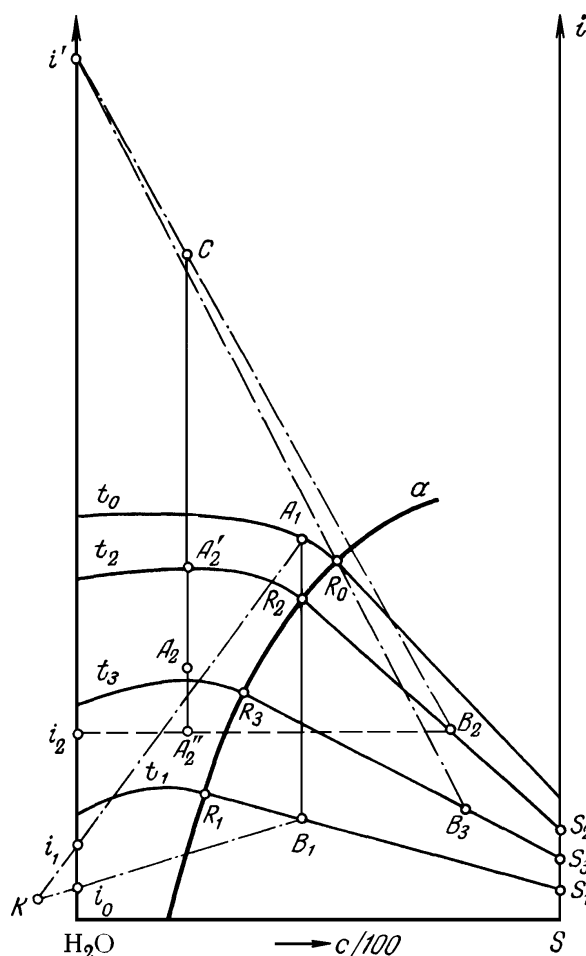
Рисунок 5.23 – Ентальпійна діаграма
