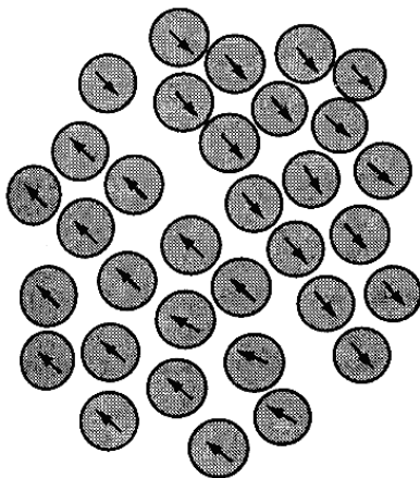
Рисунок 5.2 – Фрагмент карти розподілу скляних куль діаметром 50 мкм, суспензованих в ізотермічній нерухомій в'язкій рідині ( \mu = 0,50 Па·с, T = (296 \pm 1 К, частка об'єму, що припадає на кулі, дорівнює 0,3) , за швидкостями руху (стрілками зазначено напрям руху)
