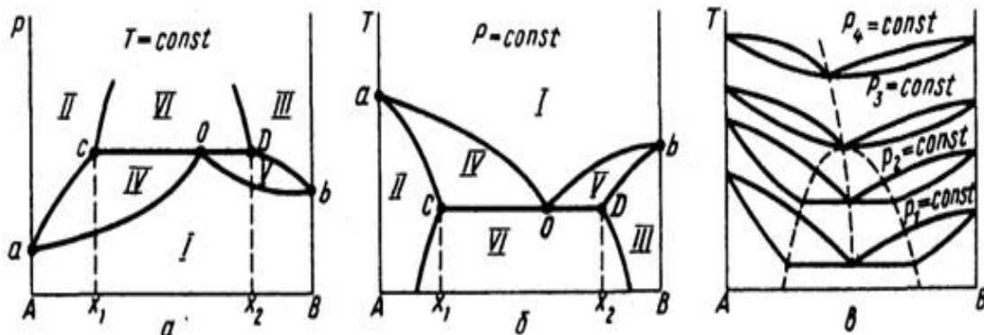
Рисунок 1.6 – Рівновага пара-рідина в системах з обмеженою взаємною розчинністю рідин ( P_1 < P < P_2 )
