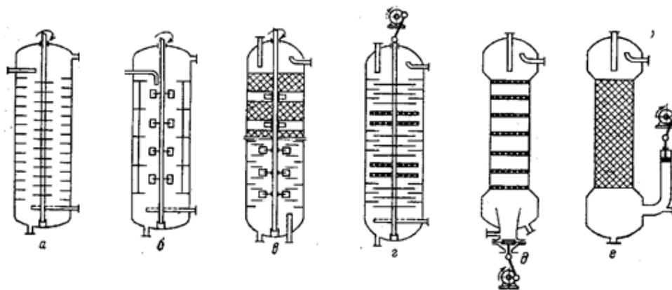
а – роторно-дисковий екстрактор; б – колона «Мікско»; в – колона Шейбеля (1 – з шарами насадки; 2 – з капсульованими мішалками); г – вібраційна колона; д – пульсаційна ситчаста колона; е – пульсаційна насадкова колона Рисунок 4.12. – Колонні апарати з механічними пристроями перемішування
