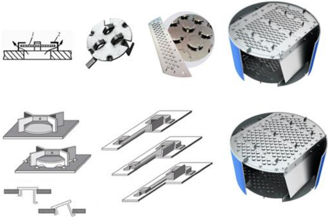
Рисунок 2.17. – Схема роботи клапана та вигляд елементів клапанної колони
