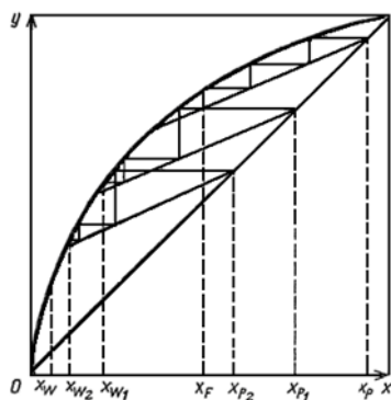
Рисунок 1.22 – Визначення складів кубової рідини, що відповідають різним значенням складів дистилятів X_{W1}, X_{W2}, \dots для заданої кількості теоретичних ступінней N_m (тут N_m = 3 )
