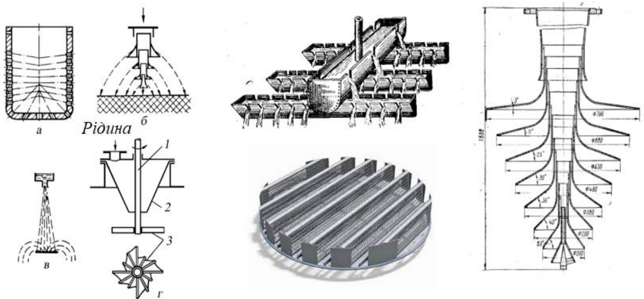
а – розподільна склянка; б – багатоконусний зрошувач; в – тарілчастий (дисковий) зрошувач; г – відцентровий розбризкувач, що обертається; 1 – вертикальний вал; 2 – напрямний конус; 3 – зірочка
