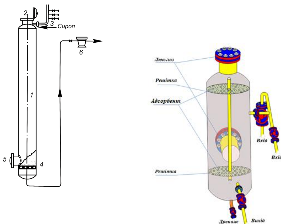
Рисунок 3.5 – Колонний адсорбер
