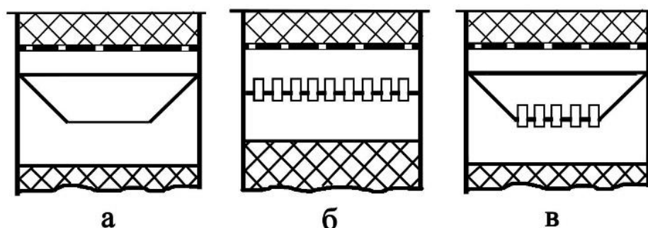
a – конічний, б – патрубковий, в – конічний з патрубками Рисунок 2.8 – Перерозподільники рідини між шарами насадки
