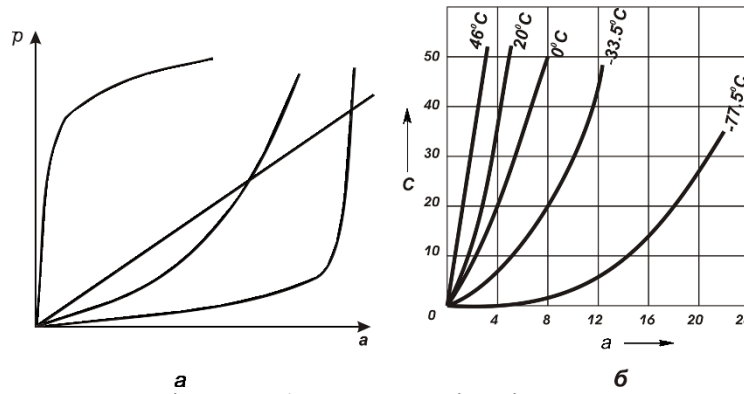
а – види типових ізотерм ( a – масова кількість поглиненої речовини, \text{кг}/\text{м}^3 ; p – парціальний тиск пари поглинається речовини, \text{мм рт. ст} ); б – ізотерми адсорбції окису вуглецю на вугіллі для різних температур ( C – концентрація окису вуглецю в газовій суміші, \text{ммоль}/\text{л} ; a – кількість поглиненого окису вуглецю, \text{ммоль}/\text{г} поглинача)
