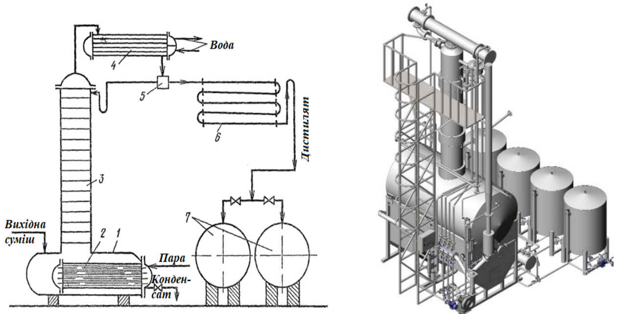
1 – куб-кип'ятильник; 2 – підігрівач; 3 – колона ректифікації; 4 – дефлегматор; 5 – дільник потоку; 6 – холодильник; 7 – збірники
