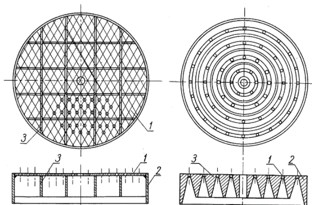
1 – тарілка; 2 – бортик; 3 – перегородки Рисунок – 4.11. Тарілка ситчаста
