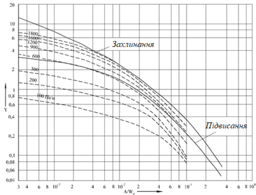
Рисунок 2.11 – Залежності для визначення швидкості газу та опору зрошуваної насадки
