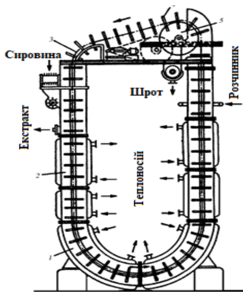
1 – кругла ділянка; 2 – вертикальна колона; 3 – роликовий ланцюг; 4 – рамки; 5 – привідний барабан Рисунок 4.31 – Дифузійний апарат безперервної дії типу J
