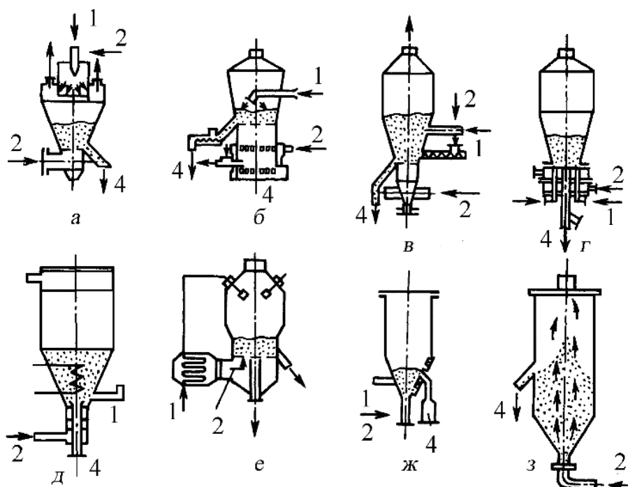
Рисунок 5.17 – Типові конструкції випарних кристалізаторів із псевдозрідженим шаром
