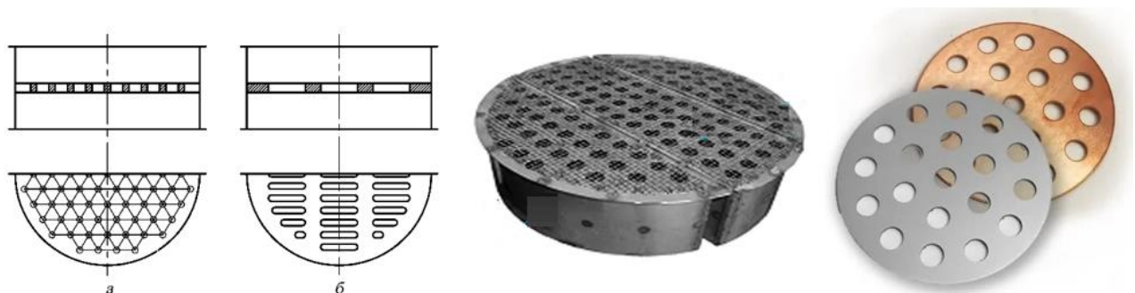
Рисунок 2.18 – Провальні тарілки
