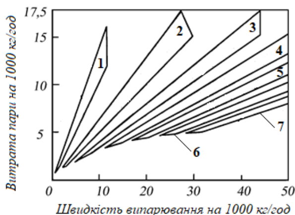
Рисунок 5.11 – Відносна витрата пари в багатокорпусних випарних кристалізаційних установках
