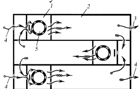
1 – камера змішування; 2 – камера відстоювання; 3 – легка фаза; 4 – важка фаза; 5 – турбінна мішалка
