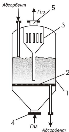
1 – корпус; 2 – газорозподільча решітка; 3 – пиловловлюючий пристрій; 4 – нижній патрубок; 5 – верхній патрубок Рисунок 3.7 – Одноступінчастий адсорбер безперервної дії з псевдозрідженим шаром
