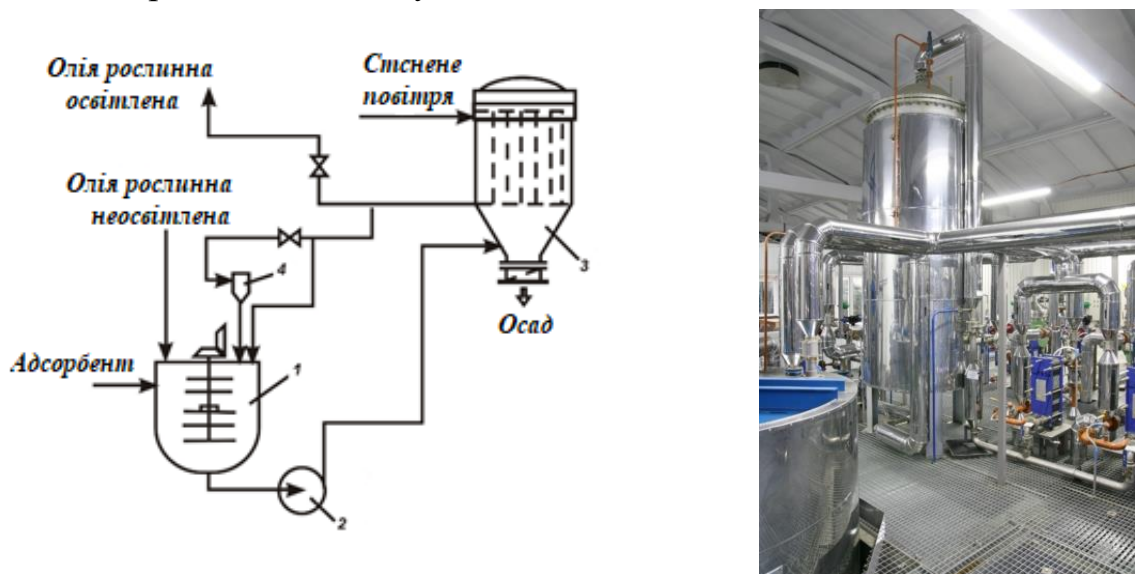
1 – адсорбер; 2 – насос; 3 – фільтр; 4 – пастка Рисунок 3.12 – Адсорбційна установка для очищення олії
