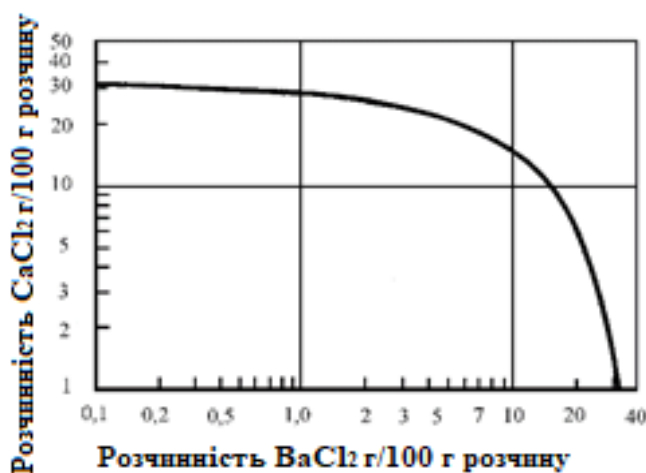
Рисунок 5.13. – Взаємна розчинність в системі \text{CaCl}_2\text{--BaCl}_2\text{--H}_2\text{O} для 50°C
