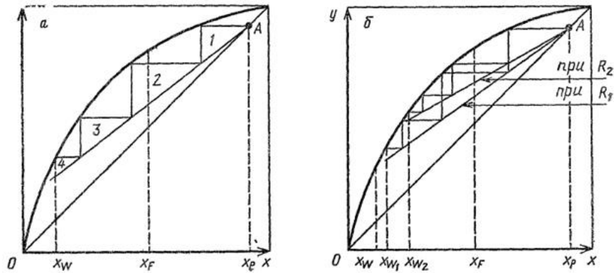
Рисунок 1.19 – Графічний метод визначення числа теоретичних ступенів Nm = 1, 2, 3 \dots зміни концентрацій (а) та складів кубової рідини x_{w1}, x_{w2}, \dots для різних значень R (б)
