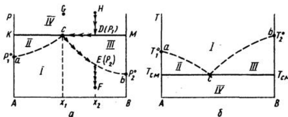
Рисунок 1.8 – Діаграма випарювання двох рідин, що не змішуються
