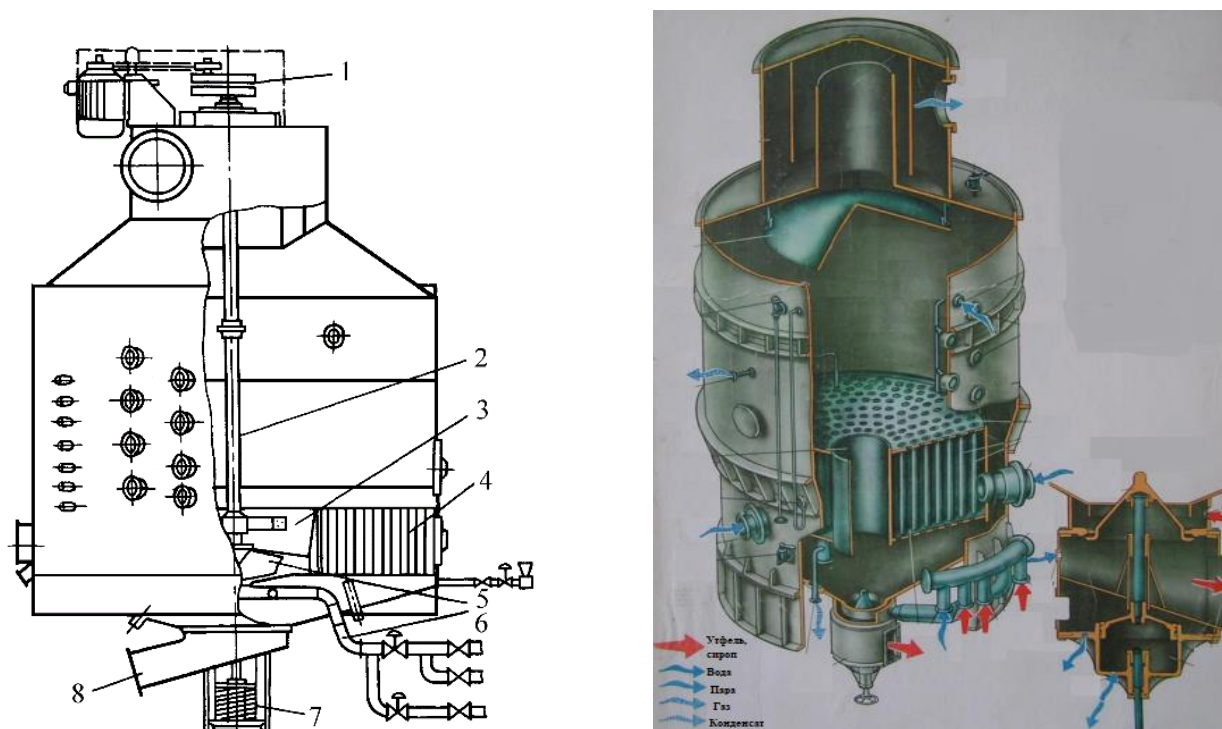
Рисунок 5.16. – Вакуум-апарат з механічним циркулятором
