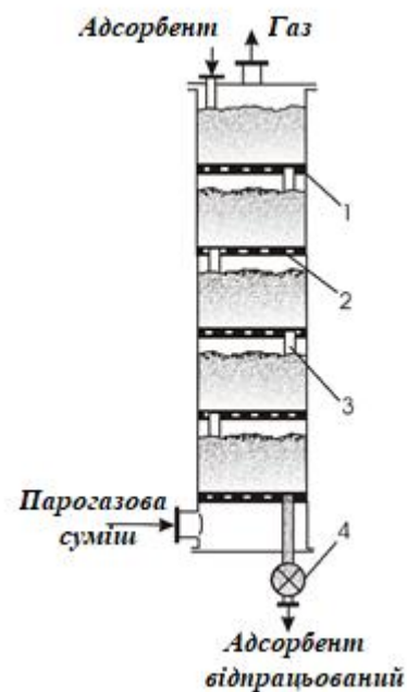
1 – корпус; 2 – газорозподільча решітка; 3 – переливний патрубок; 4 – шлюзовий затвор Рисунок 3.8 – Багатоступінчастий адсорбер з псевдозрідженим шаром
