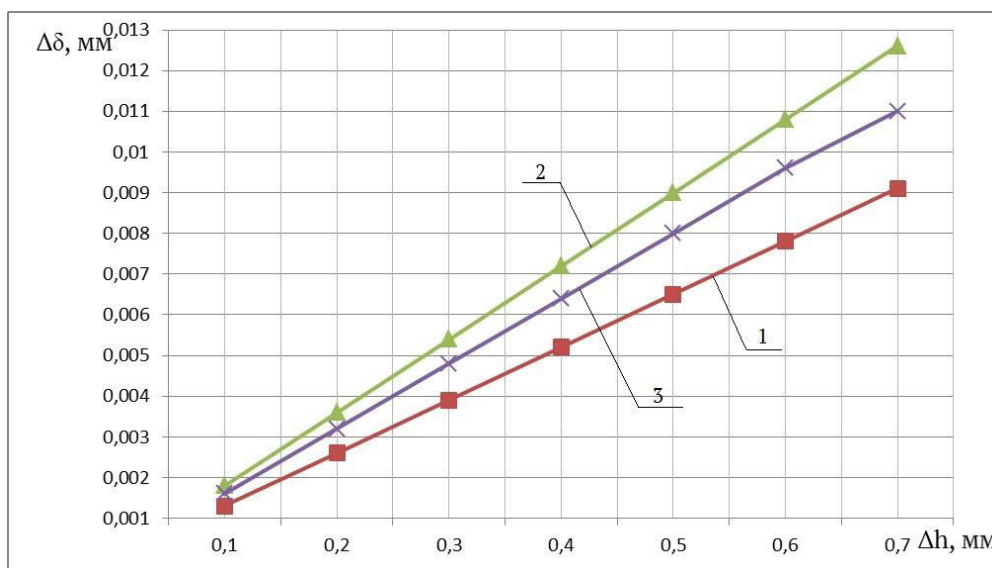
Рисунок 3 – Залежність зазору ( \Delta\delta ) у спряженні «кільцева опора п'яти – опора люльки» від зносу кільцевої опори по висоті ( \Delta h ) та тиску робочої рідини:
