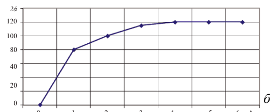
Залежність від характеристики насадки A: а – коефіцієнтів \mu і \phi ; б – кута розливу 2\alpha
