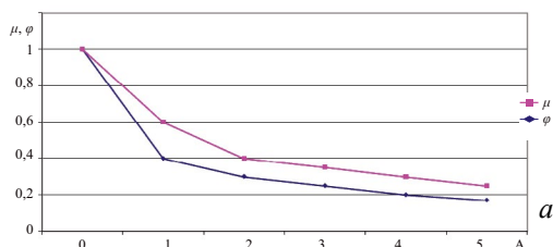
Залежність від характеристики насадки A: а – коефіцієнтів \mu і \phi ; б – кута розливу 2\alpha
