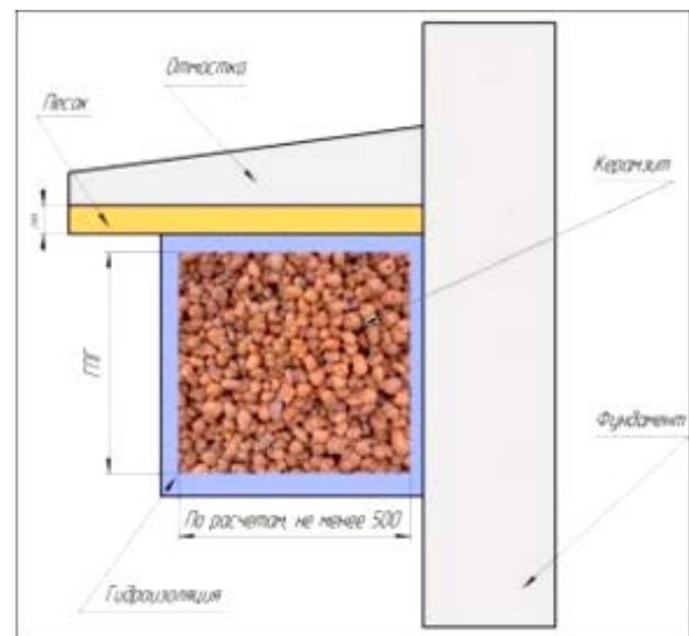
Рис. 2. Утепление фундамента керамзитом
