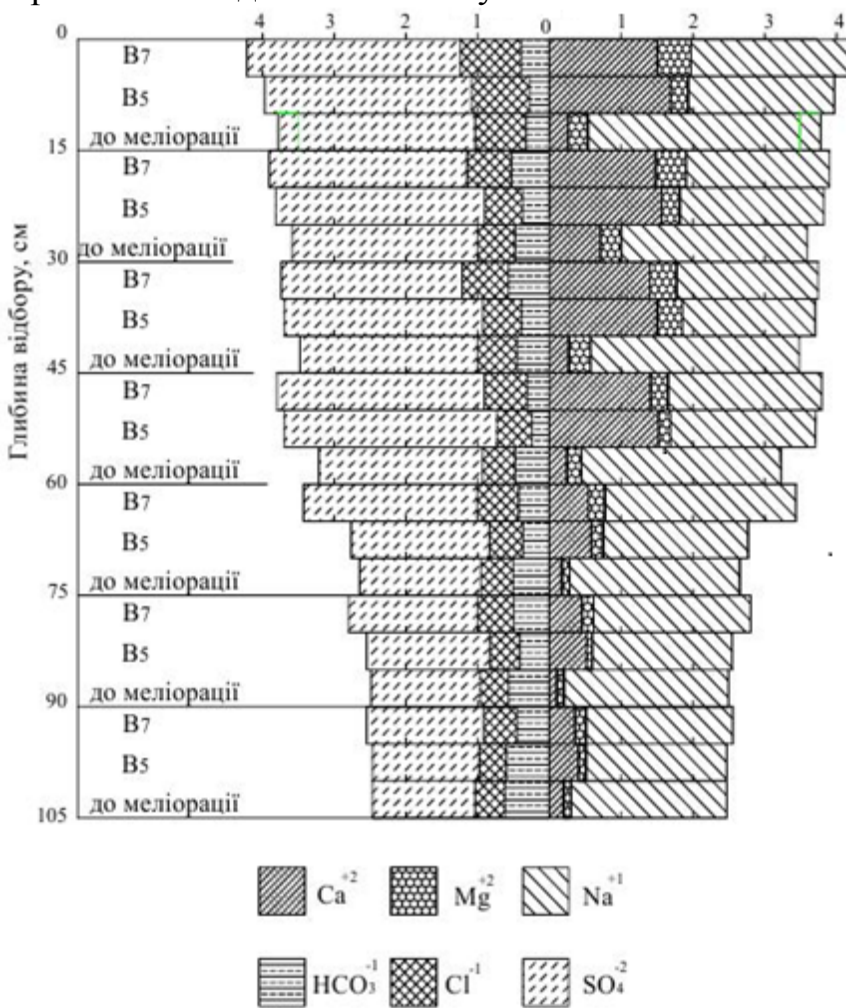
Рис. 4. Вплив фосфогіпсу при зрошенні та без поливів на сольовий профіль (третій рік післядії), мекв/100 г ґрунту
