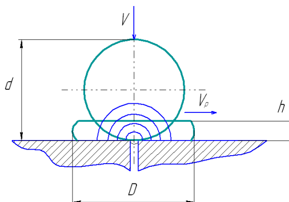
Рис. 3.13. Схема зіткнення частки змащення з підложкою
