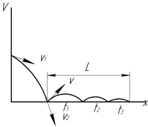
Рис 3.3 — Траекторія руху гранули
