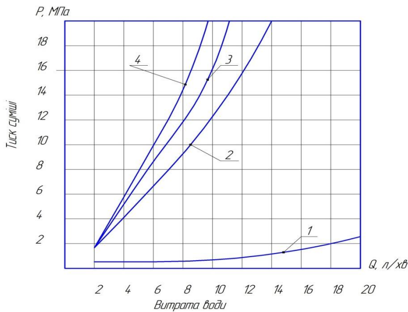
Рис. 3.9. Залежність витрати води від тиску, що створює установка
