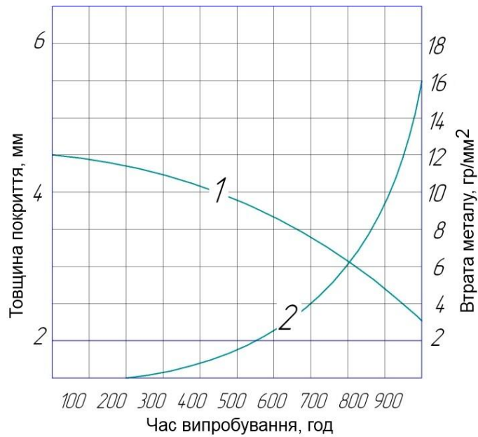
Рис. 3.17 Вплив зовнішніх кліматичних факторів на ефективність протекторного захисту «WD40+ЦП1» при багатокомпонентному захисті стикових з'єднань і щілин
