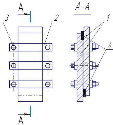
Рис. 3.15 - Пристосування для визначення проникаючої здатності рідкого протектора
