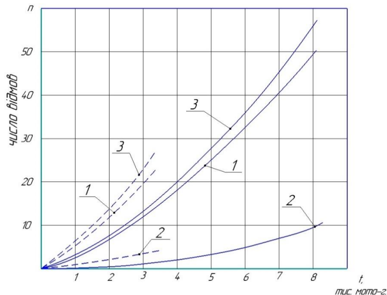
Рисунок 4.2 - Середнє накопичене число відмов тракторів модифікації МТЗ в умовах реальної експлуатації: ----- до першого капремонту; - - - - після капітального ремонту; 1 - відмови II групи складності, 2 - відмови III групи складності, 3 - сума відмов II і III груп складності.
