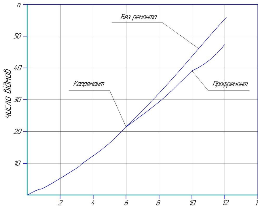
Рисунок 4.7. – Динаміка показників старіння трактора при одному капітальному і одному профілактичному ремонтах
