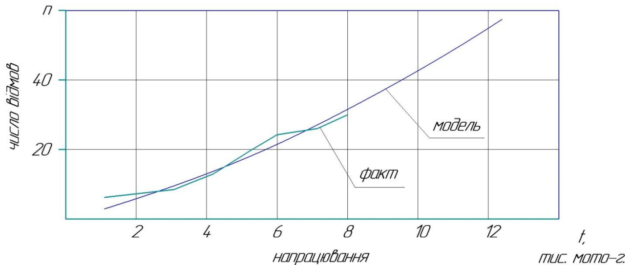
Рисунок 4.4. - Динаміка значущих (II і III групи складності) відмов
