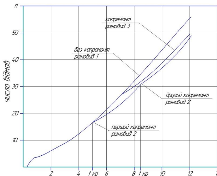
Рисунок 4.5. – Динаміка старіння тракторів з різними варіантами капітальних ремонтів
