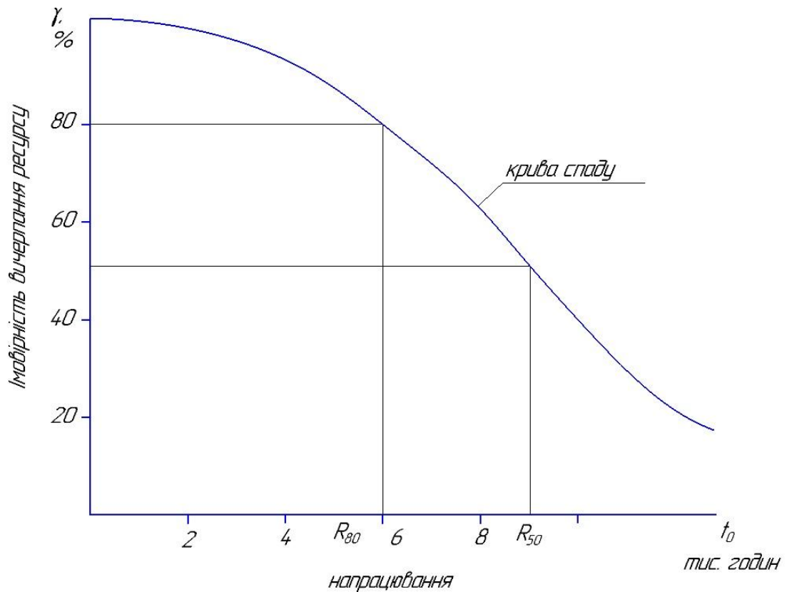
Рисунок 2.2 – Крива спаду.
