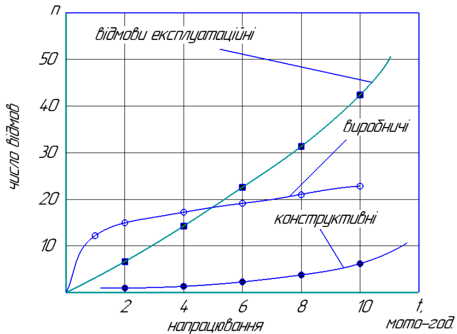
Рисунок 4.1 - Динаміка відмов з різних причин їх появи.
