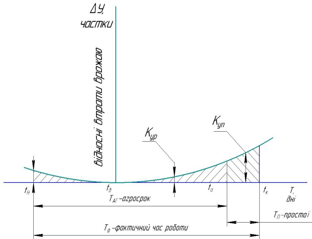
Рисунок 3.3 - Схема визначення питомих втрат врожаю при простоях комбайна
