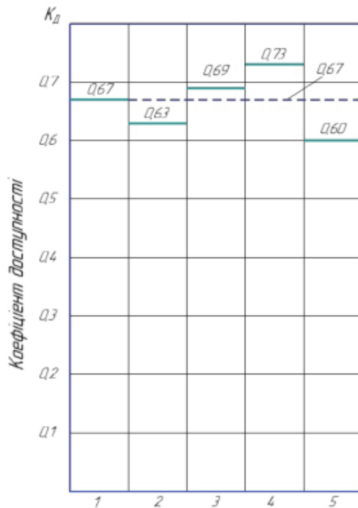
Рис.1 – Показники коефіцієнта доступності при проведенні технічного обслуговування ТО-3 для гідравлічної системи трактора ЮМЗ-8244: 1.- насос шестеренний; 2. – гідророзподільник; 3. – силовий гідроциліндр; 4. – гідравлічний бак; 5. – гідравлічні рукава.
