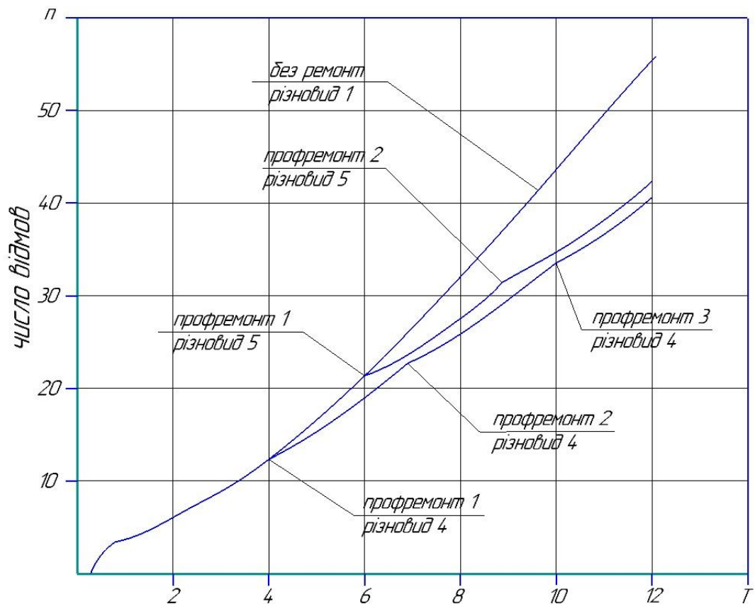
Рисунок 4.6. – Динаміка показників старіння тракторів з різними варіантами профілактичних ремонтів.
