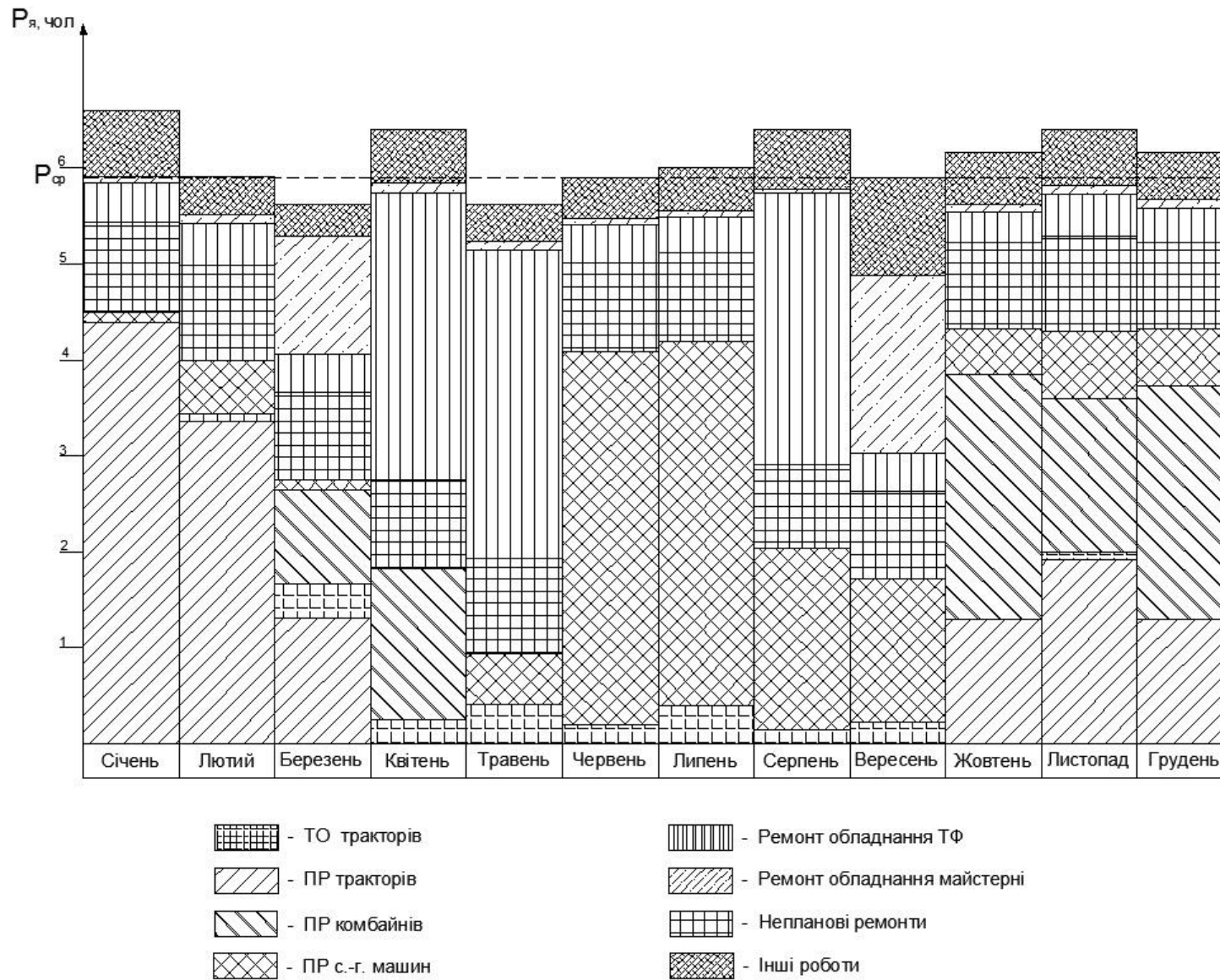
Рис.4.8 – Річний графік завантаження майстерні
