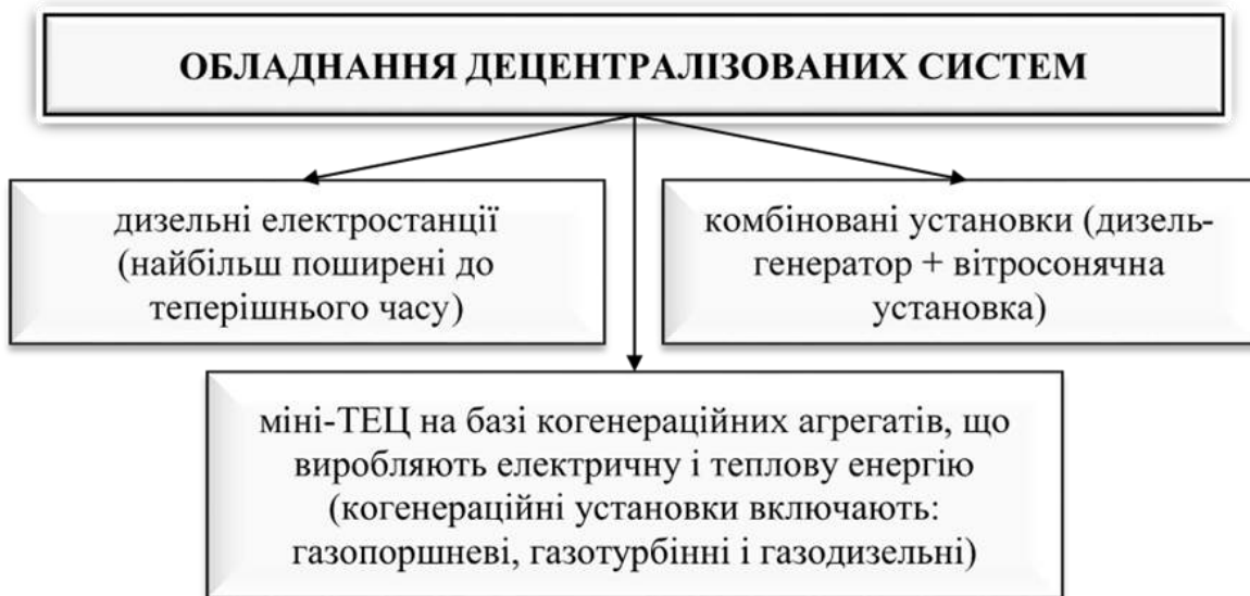
Рисунок 1. Енергетичне обладнання децентралізованих систем
