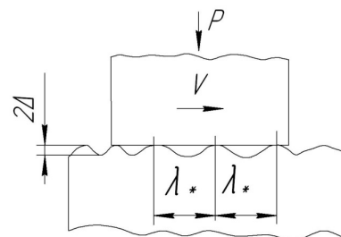
Рисунок 1 – Схема взаємодії шорстких поверхонь для розгляду механізму термопружної нестійкості
