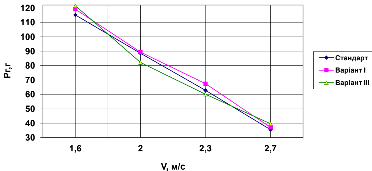
Рисунок 4.8 - Залежність маси ґрунту, що налипає на культиваторних лапах в залежності від швидкості руху при міжрядному обробітку
