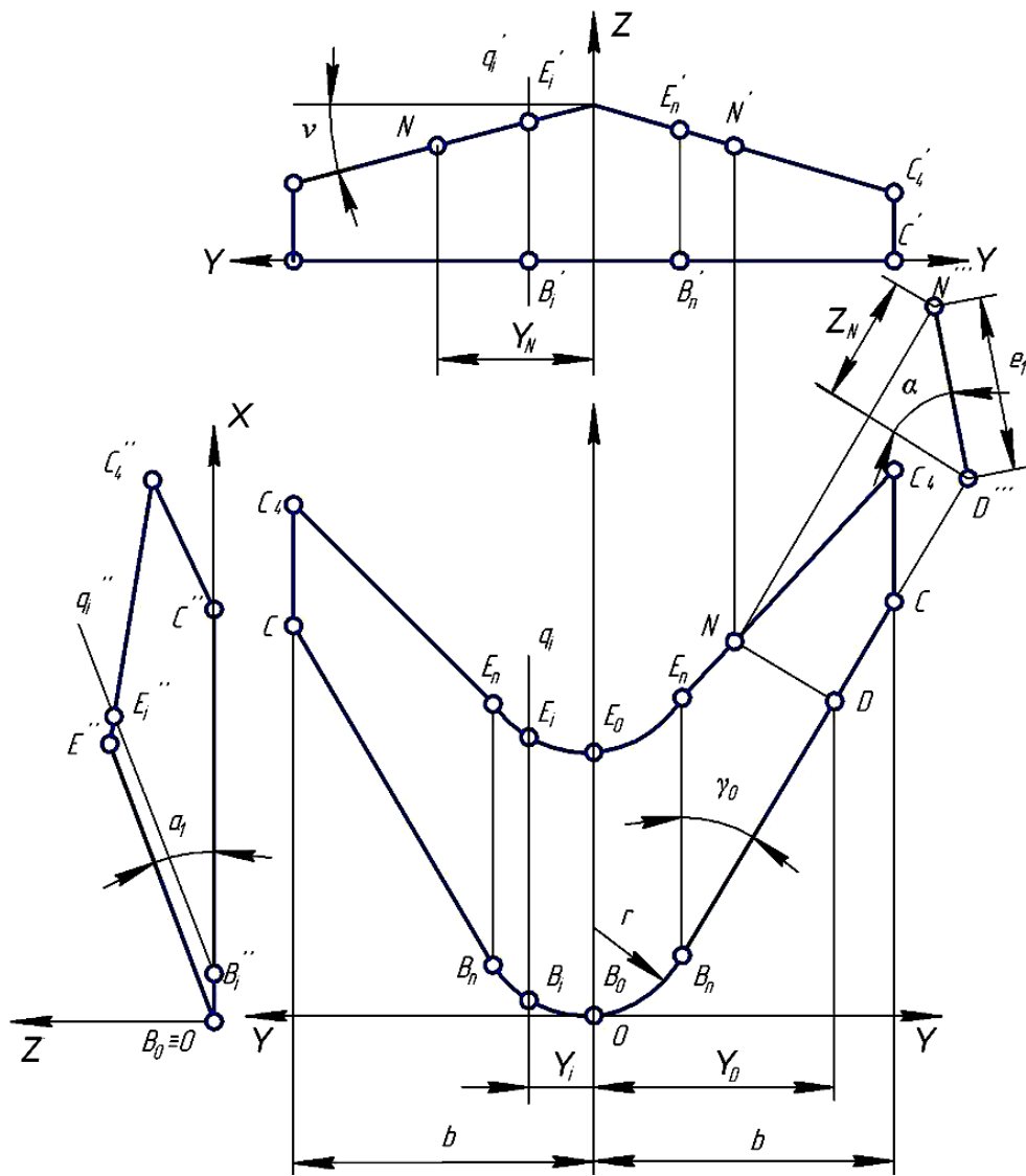
Рисунок 2.8 - Схема побудови поверхні лапи
