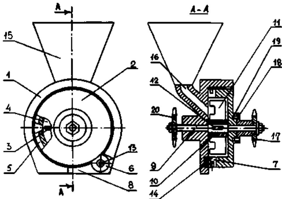
Рис. 3.2. Висівний апарат:
