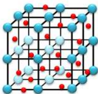
Рис. 4.11. Металічний зв'язок:
