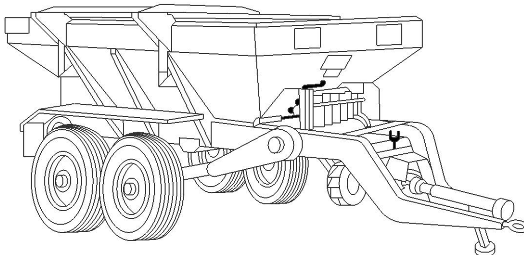
Рис. 2.3 Машина СТТ-10
