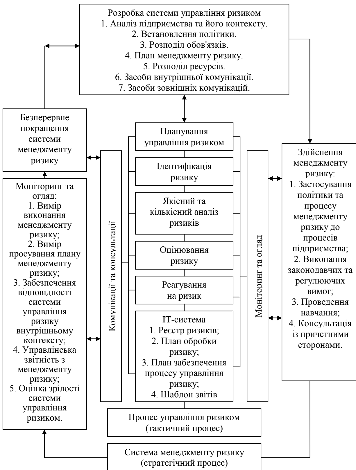
Рис. 3.4. Алгоритм управління ризиками на підприємствах
