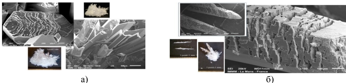
Рис. 2. – Кристали гіпсу, вирощені з добавкою: а) – Master X-Seed 100; б) Sika.
