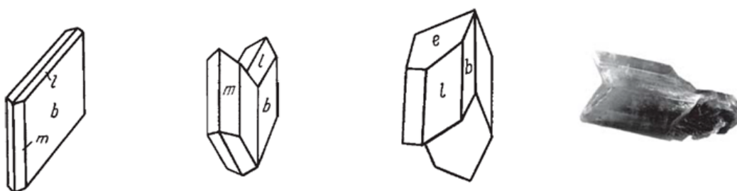
Рисунок 2 – Кристали гіпсу : а) кристал гіпсу у вигляді пластини: b \{010\} , l \{111\} , m \{110\} ; б) гальський двійник зростання по (100): m \{010\} , l \{111\} , b \{010\} ; в) парижський двійник зростання по (101): l \{111\} , b \{010\} , e \{103\} ; г) хвіст ластівки – прозорий двійник гіпсу.
