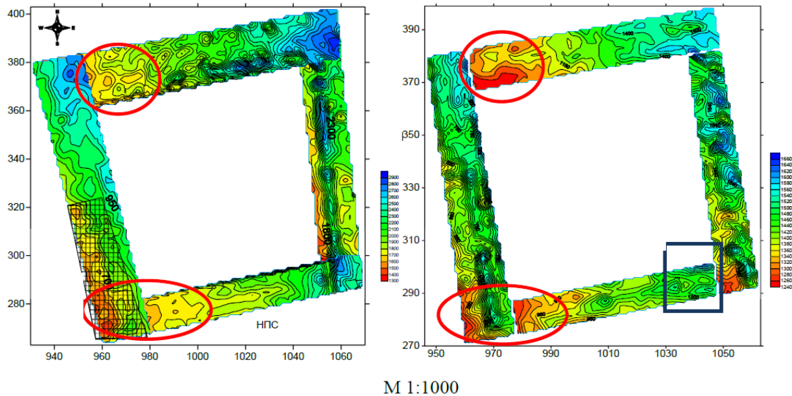
Рисунок 1 – Карти-схеми щільності потоку імпульсів магнітної складової ПЕМПЗ за антенами схід-захід у різні роки спостережень: а) 2013 р.; б) 2017 р.; 1, 2, 3 – ділянки фільтрації.
